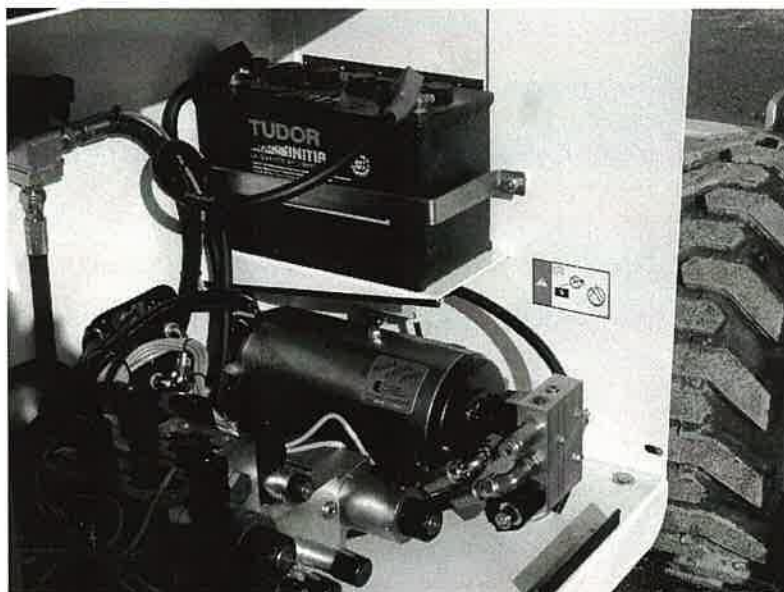
Foto 16 - Generatriz embarcada
