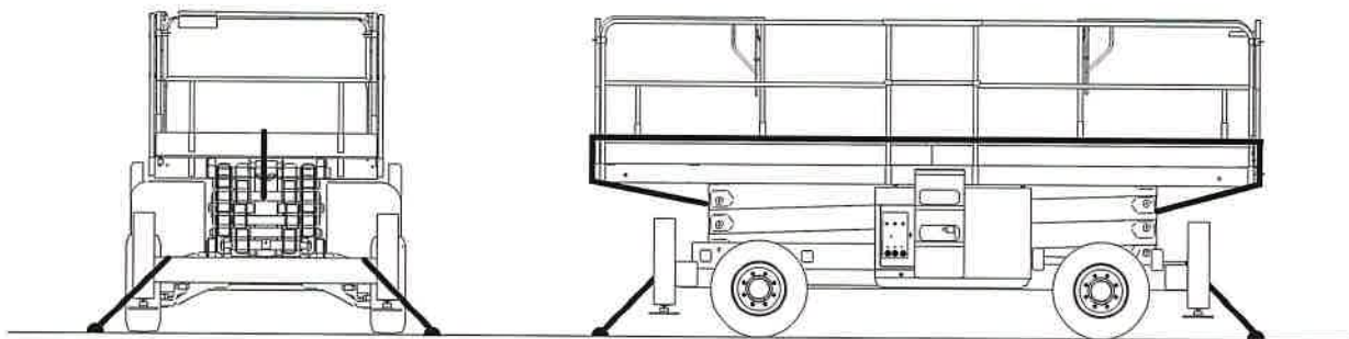
Dibujo : Disposición y sujeción de la carga
